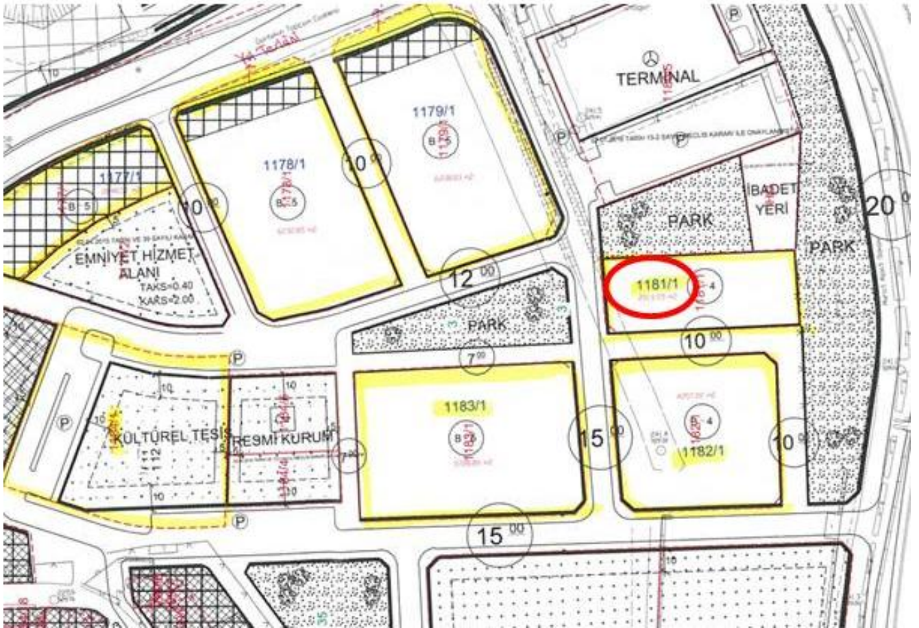
1/1.000 Ölçekli Uygulama İmar Planı
