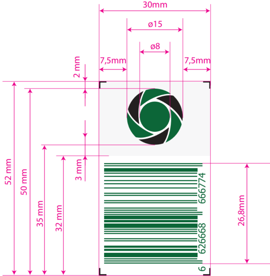
Şekil 4 Alüminyum Ambalaj Kutu için DYS İşareti ve Ölçüleri
