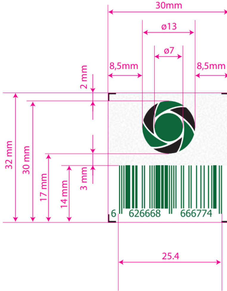
Şekil 3 Alüminyum Ambalaj Kutu Harici DYS İşareti ve Ölçüleri
