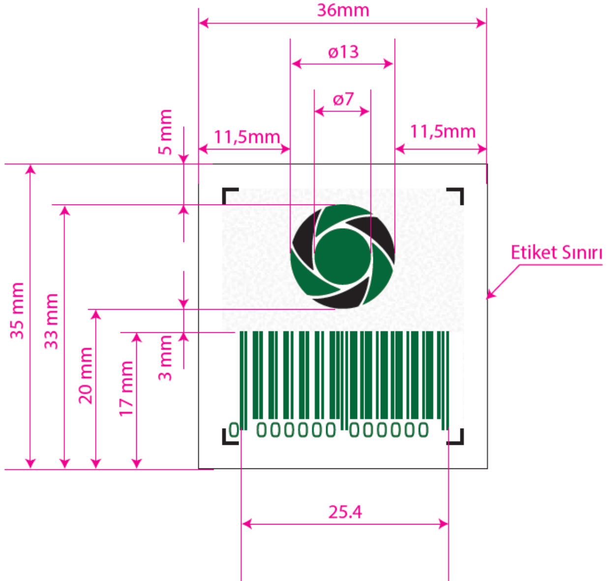
Şekil 10 Yapışkanlı DYS Etiket Ölçüleri
