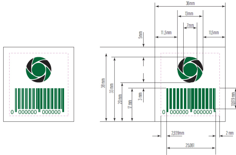
Şekil 5 Yapıştırma DYS Etiket Ölçüleri
