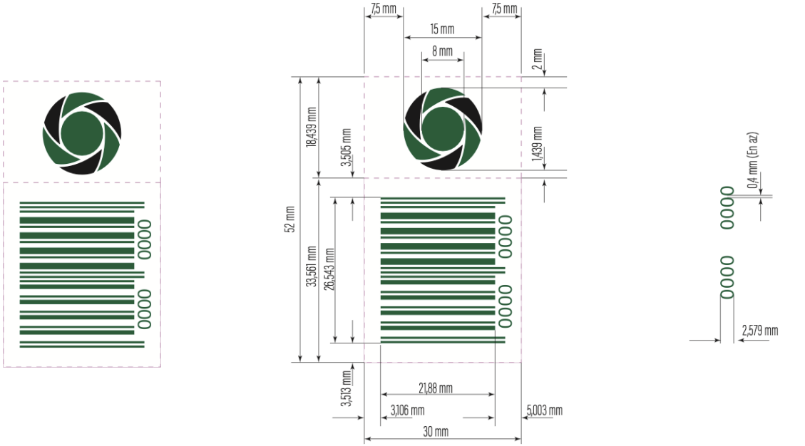
Şekil 4 Alüminyum Kutu Ambalaj ve Shrink Sleeve Etiket DYS İşareti ve Ölçüleri
